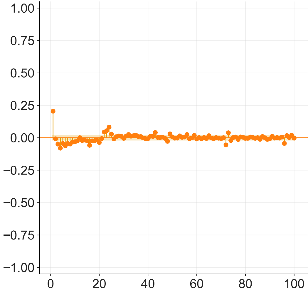
PACF MSM (2022)
